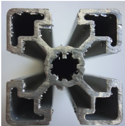
Werkstück vor dem Bürstvorgang
